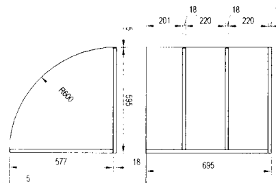
C - Rohová skříňka - 1ks
