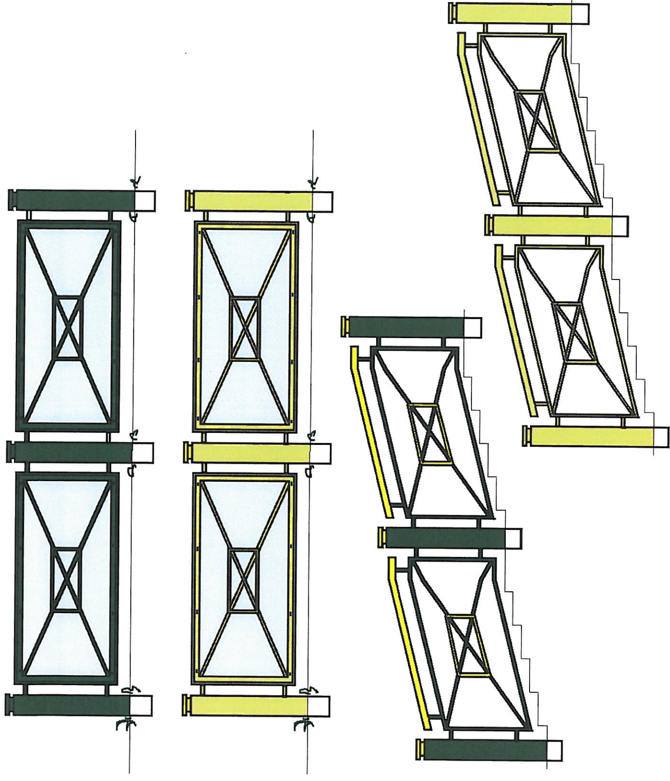
Varianta "A" s vloženým polykarbonátem a různém barevné provedení
