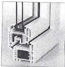
ALUPLAST Ideal 4000 5k, 70 mm, předsazené křídlo
