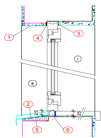
Detail osazení okna 1:5
