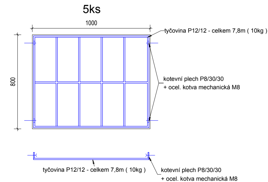
Mříž Z2 ( 1:20 )
