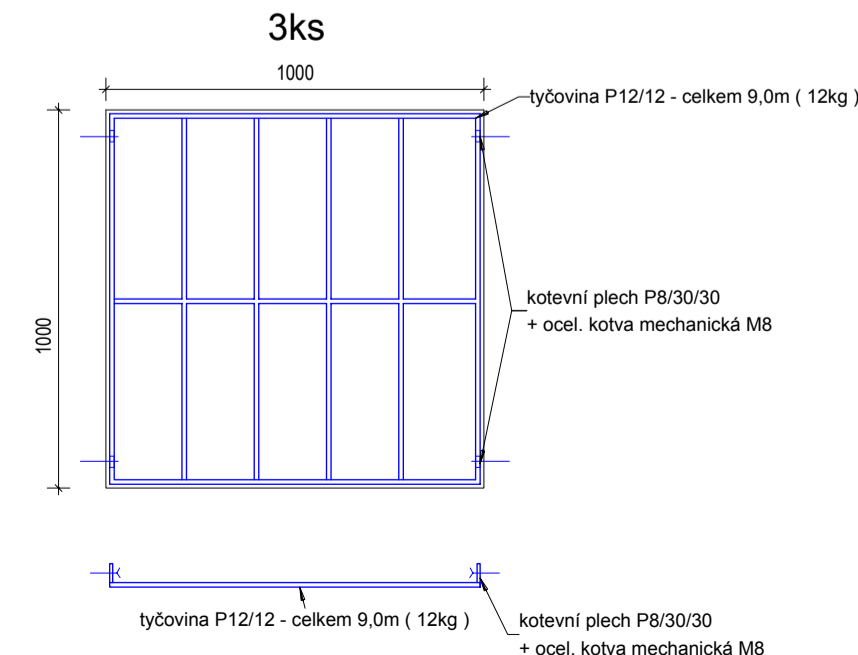
Mříž Z3 ( 1:20 )
