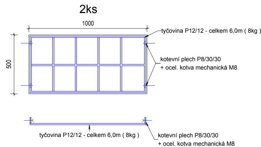
Mříž Z1 ( 1:20 )
