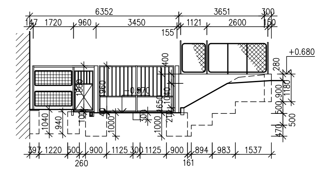
POHLED B-B 1:100
