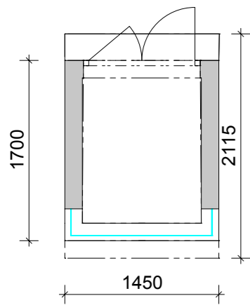
objekt prodeje lístků M 1:50
