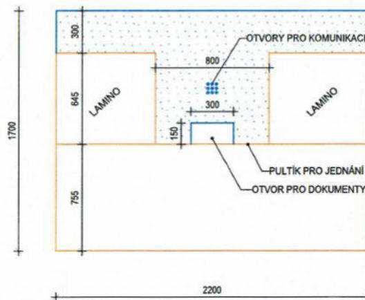
POHLED A
