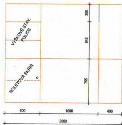
POHLED C
