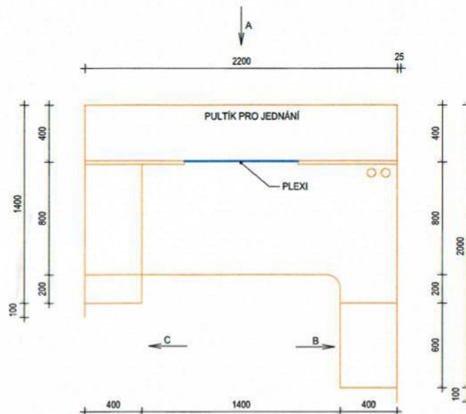
POHLED A
