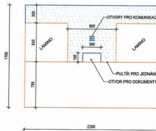
POHLED A
