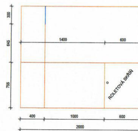
POHLED B
