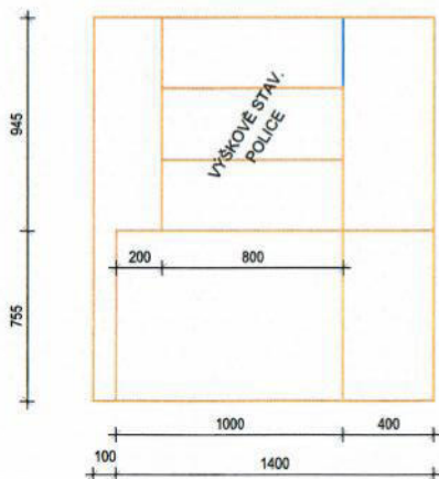
POHLED C
