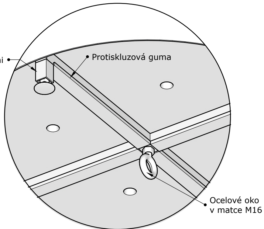
Detail řešení konstrukce dna
