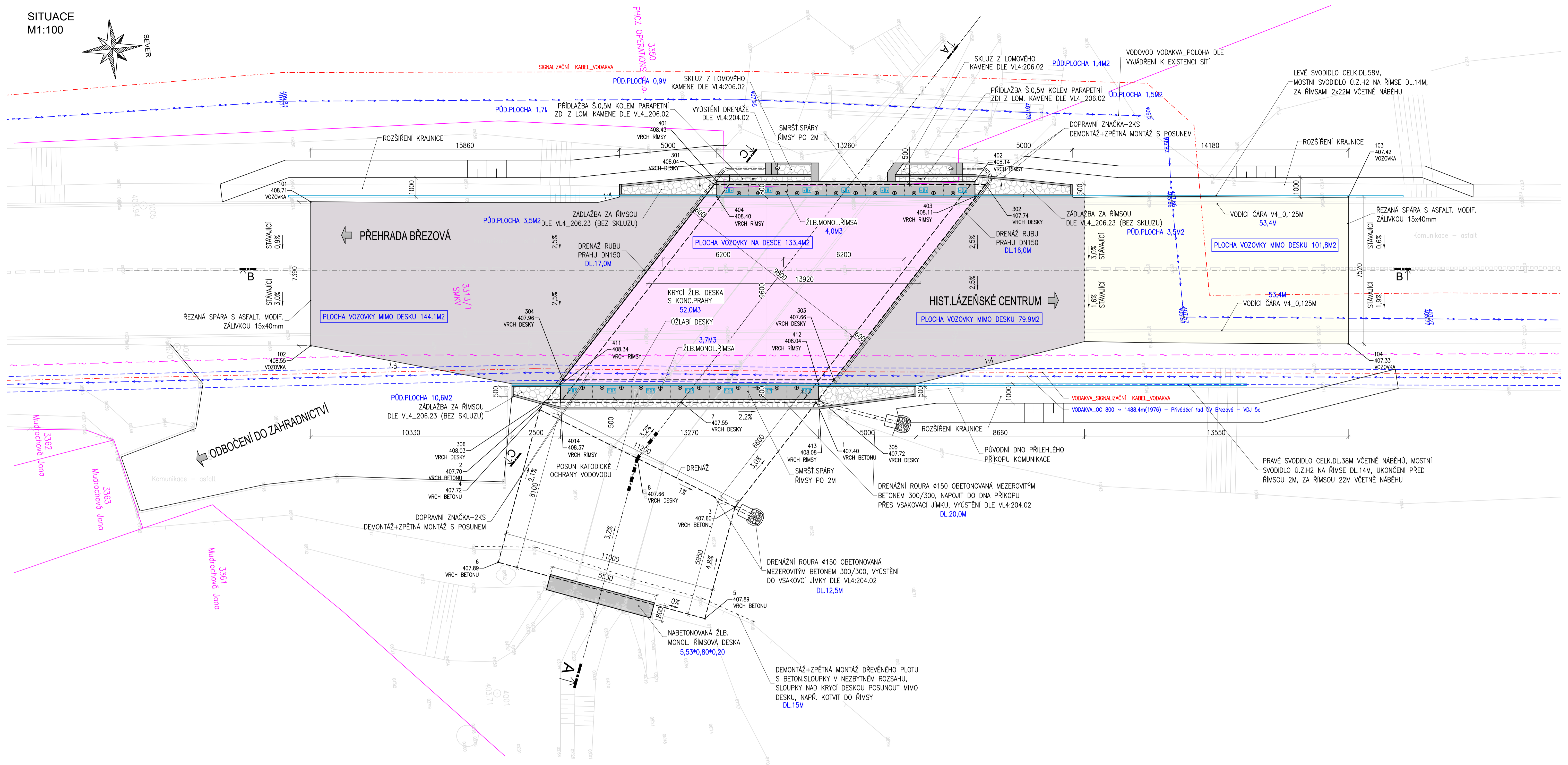
ROHY ROZSAHU ÚPRAVY VOZOVKY
