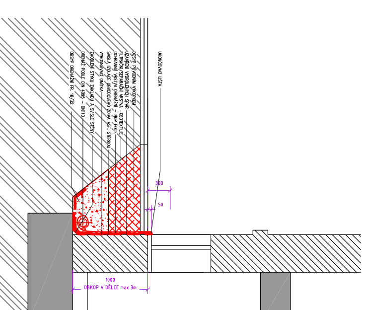
ŘEZ 1-1 - NOVÝ STAV, M1:50
