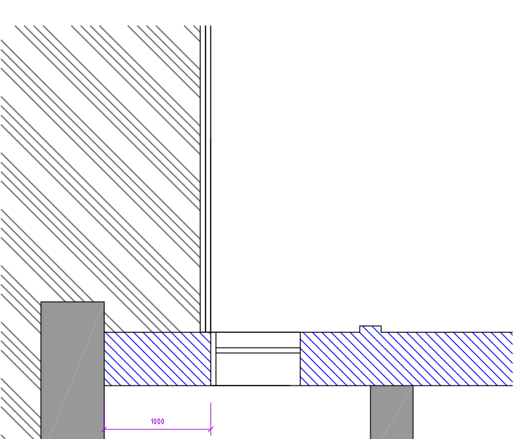
ŘEZ 1-1 - STÁVAJÍCÍ STAV, M1:50
