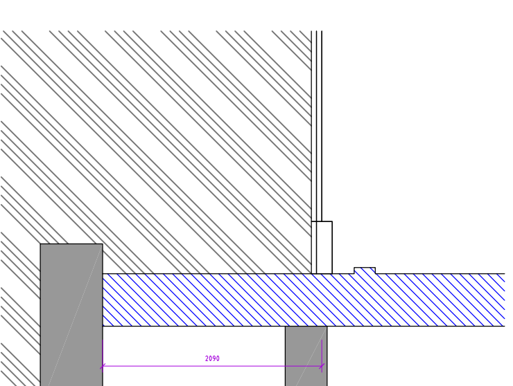
ŘEZ 2-2 - STÁVAJÍCÍ STAV, M1:50
