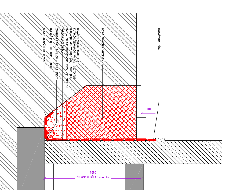
ŘEZ 2-2 - NOVÝ STAV, M1:50
