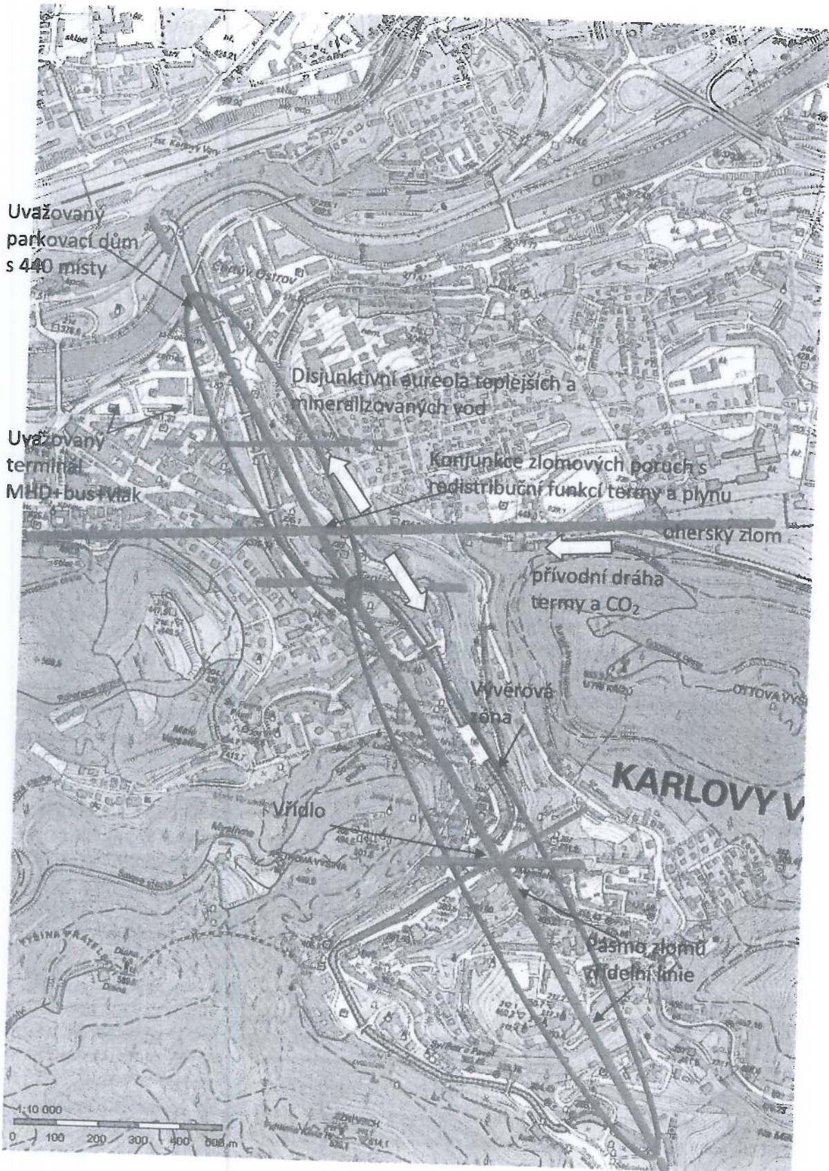
Obr. 1 Orientační mapa se základním tektonickým schématem
